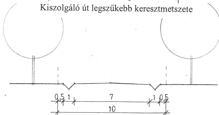
Külterületi vegyesforgalmú kiszolgáló út (dülőút) legszűkebb keresztmetszete
