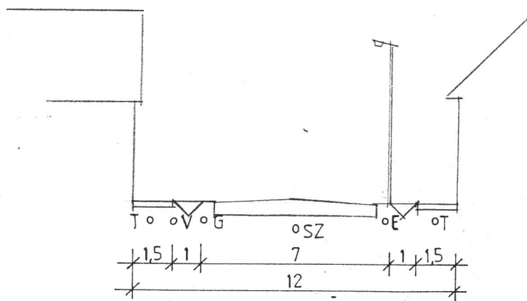
Kiszolgáló út legszűkebb keresztmetszete
