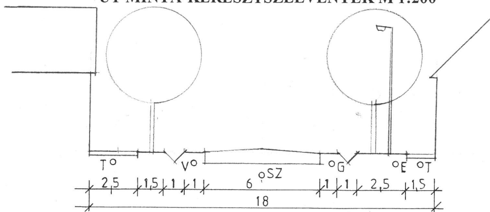
Országos mellékút (Kossuth u.) legszűkebb keresztmetszete
