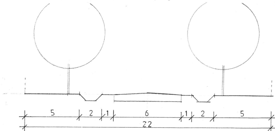
Tervezett gyűjtőút legszűkebb keresztmetszete
